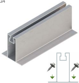
Perfil G4
